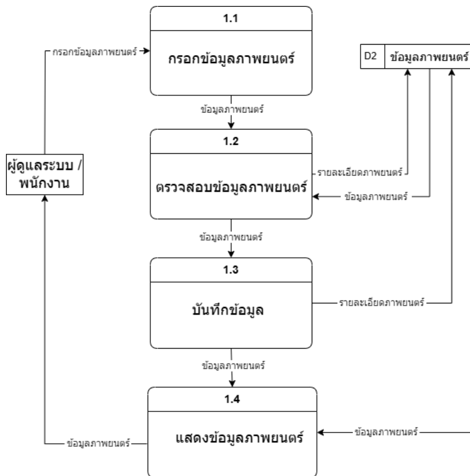
ภาพที่ 3.5 แผนภาพ DFD Level 2 โพรเซสที่ 1 เพิ่มข้อมูลภาพยนตร์
