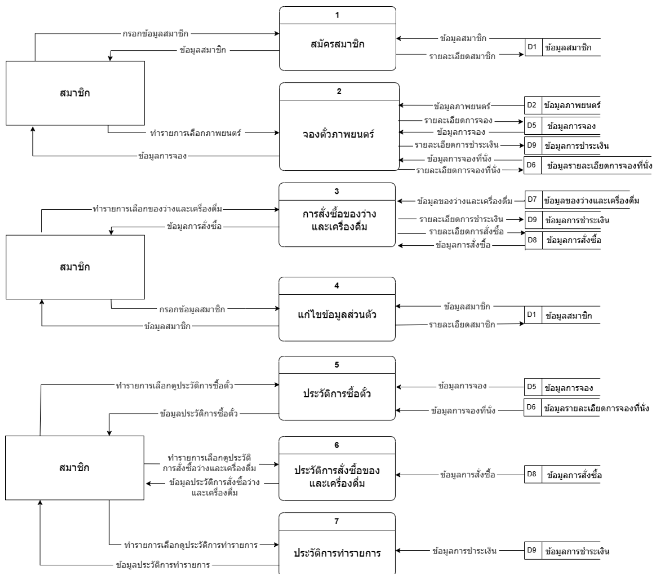
ภาพที่ 3.4 แผนภาพ DFD Level 1 ส่วนของสมาชิก
